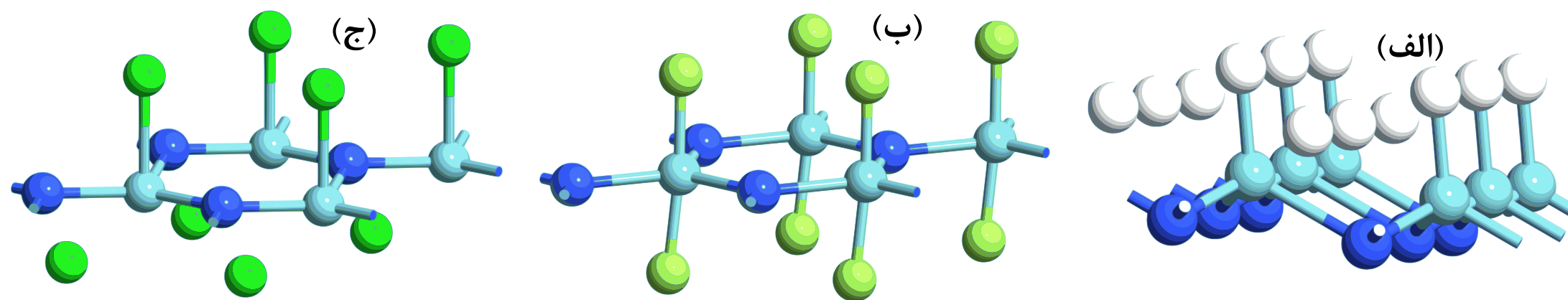
شکل 1: الف) ساختار اتمی 2x3 تکرار شده پس از بهینه سازی و جذب اتم هیدروژن در راستای y-z (ب) جذب فلور (ج) جذب کلر. هر یک از ساختارها 4 اتم در یاخته واحد خود دارد. اتم H, F, و Cl به ترتیب با گوهای سفید، سبز کم رنگ و پر رنگ نشان داده شده اند.
