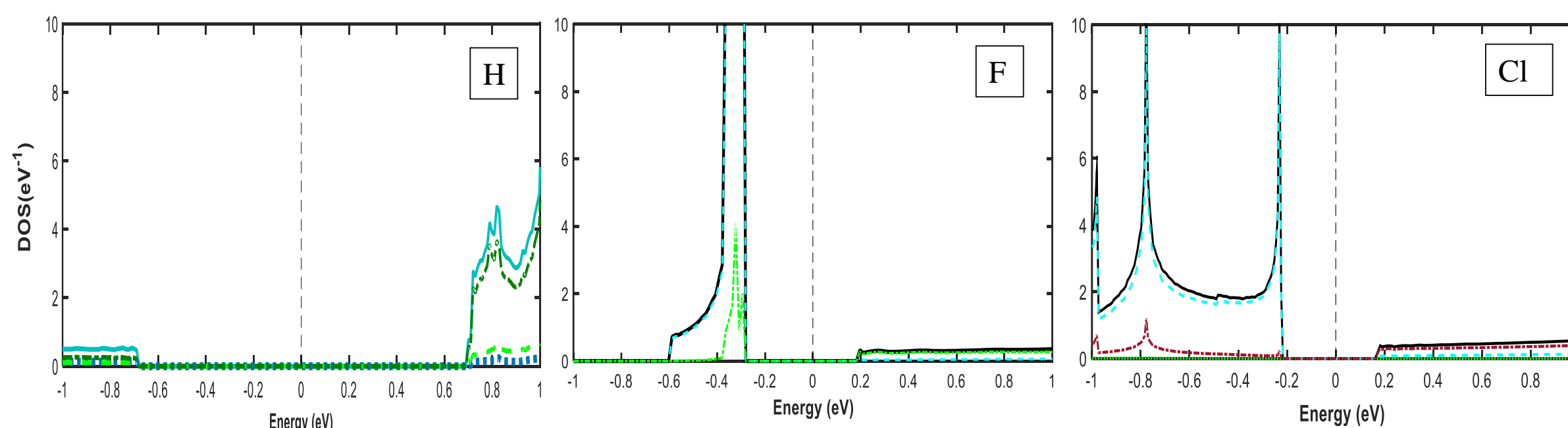
شکل 3: چگالی حالت ها پس از جذب ناشی از اوربیتال های اتمی. اوربیتال d در جذب H به رنگ سبز پر رنگ و اوربیتال p در جذب F و Cl به رنگ آبی روشن است.
